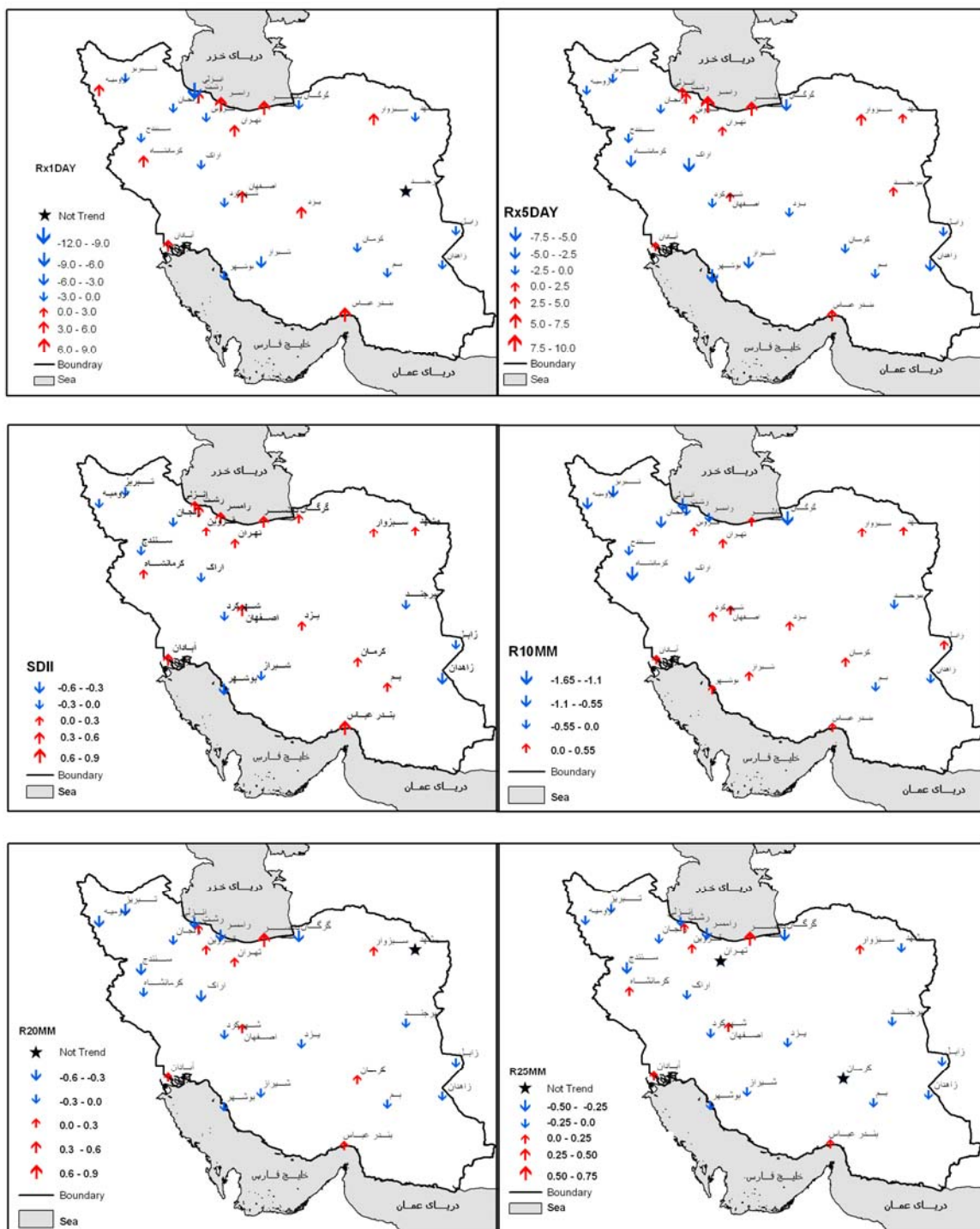
شکل ۱- روندهای خطی نمایه‌های حدی بارش در دوره ۲۰۰۳-۱۹۵۱.
