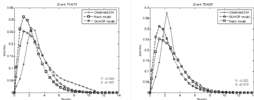
شکل ۴ - نمودار مرحله صحت سنجی مدل‌های GUHCR و Nash
