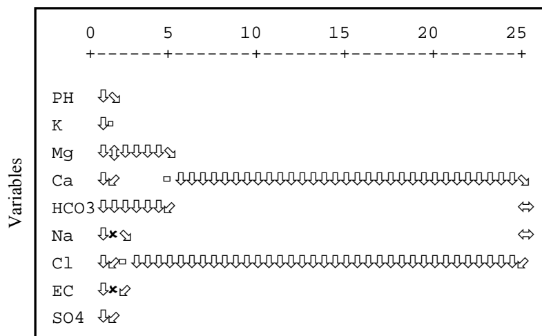
شکل ۶- نمودار تحلیل خوشه‌ای متغیرهای کیفیت آب زیرزمینی دشت کرمان
