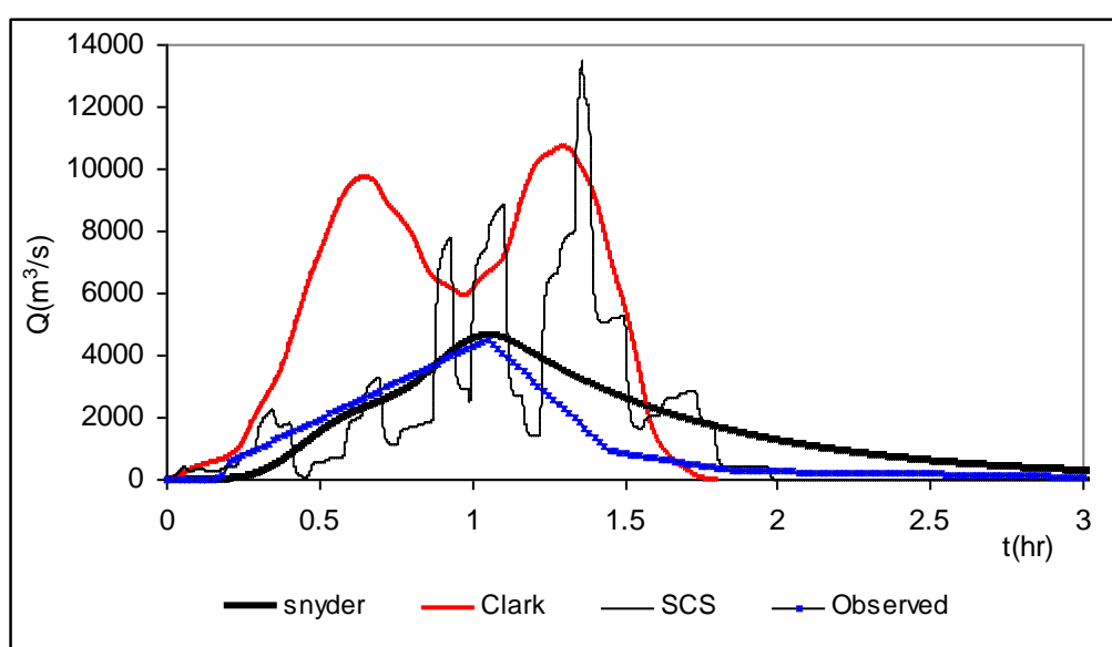
شکل ۱ - هیدروگراف‌های مشاهده شده و شبیه‌سازی شده با روش‌های اشنايدر، کلارک و SCS
